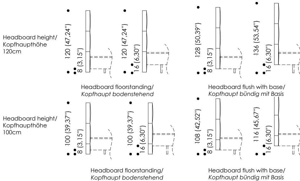
Figure with Wittmann standard foot heights/ Abbildung mit Wittmann Standardfußhöhen
