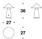
TRL (33) LAMPADA DA TAVOLO NOTTE / BEDSIDE TABLE LAMP Ø 27x36H.cm Ø 10 3/4x14 1/4H."
