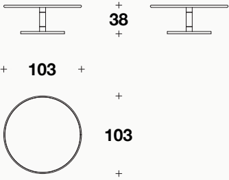
SIDE TABLE: CTD (25G) L-D= Ø 103 (Ø 40 2/3") H= 38 (15")
